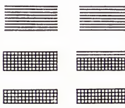
Рис. 1. Заполнение энергетических зон при абсолютном нуле температуры: а — в диэлектриках; б — в металлах; разрешённые зоны заштрихованы, заполненные зоны или их части заштрихованы дважды.
